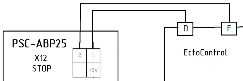
Схема подключения кнопки "Стоп" к Эктоконтрол
