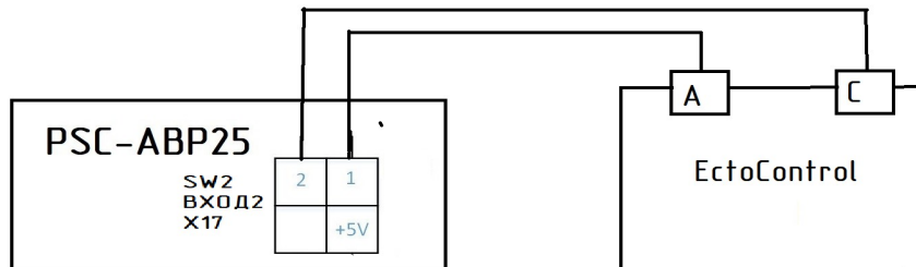
Схема подключения EctoControl как комнатный термостат
